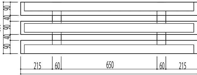
↑A側 平面図 1 / 10
