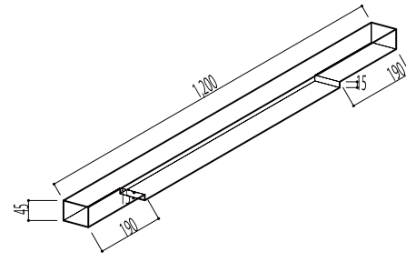
平板受け材×3本
