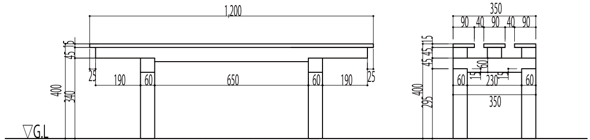
A側立面図 1 / 10
